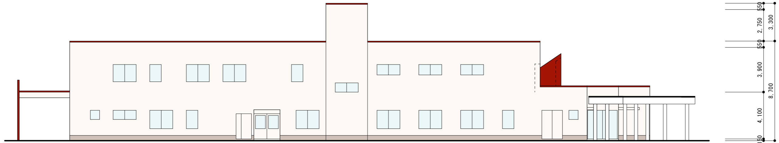
北面 立面图
